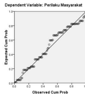
Gambar 1 Normalitas Data
