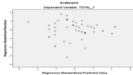
Gambar 4. Grafik Scatterplot
