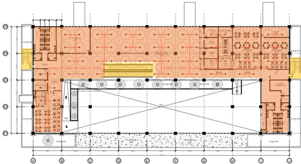
1 GAMBAR 23 Denah sistem proteksi kebakaran pada bangunan terminal penumpang
