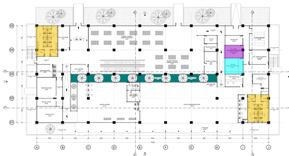
GAMBAR 14 Denah toilet lantai dasar bangunan terminal penumpang
