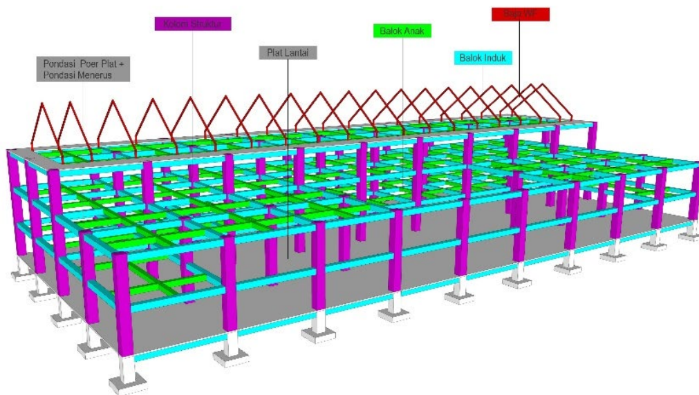
GAMBAR 22 Sistem struktur pada bangunan terminal penumpang
