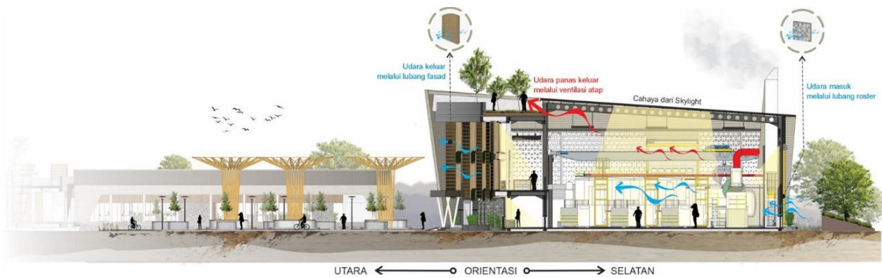
Gambar 4. Skema Penghawaan dan Pencahayaan Alami Pada Bangunan
