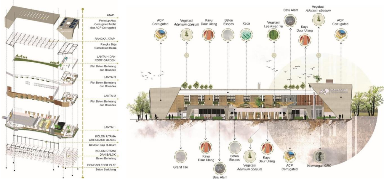
Gambar 6. Struktur Bangunan Utama dan Material Elemen Fasad
