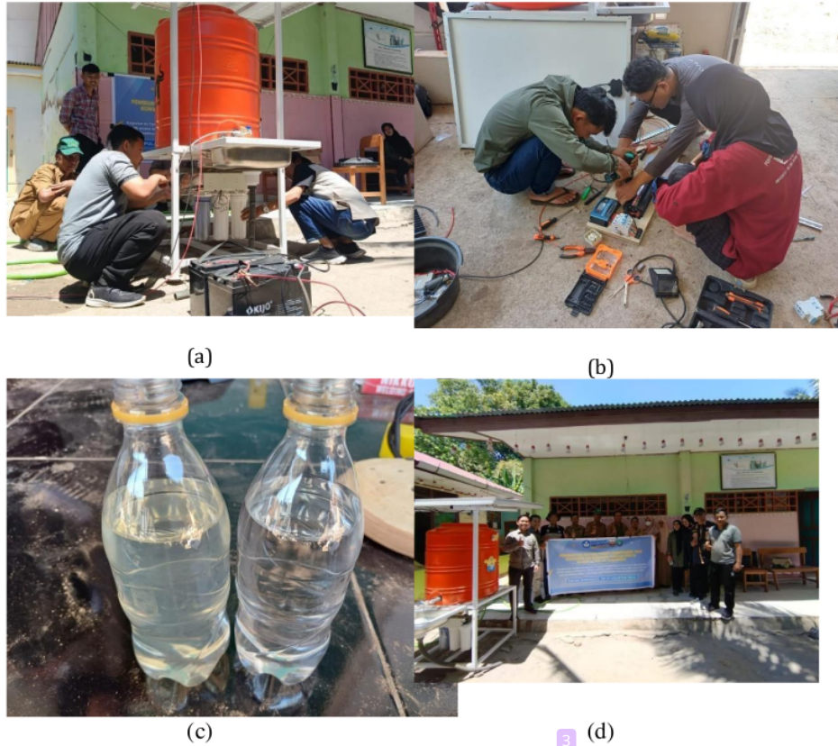
Gambar 2. Beberapa dokumentasi pelaksanaan PKM. (a) instalasi sistem pompa submersibel dan konversi air layak konsumsi berbasis tenaga surya, (b) instalasi KIT pembangkit listrik tenaga surya, (c) tampilan hasil pengujian sistem pompa submersibel dan konversi air layak konsumsi berbasis tenaga surya, (d) serah terima bahan, alat dan inovasi/ produk kepada UPT SDN 41 Sabangko
