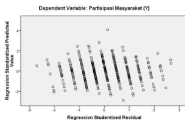
Gambar 2. Uji Heteroskedastisitas
