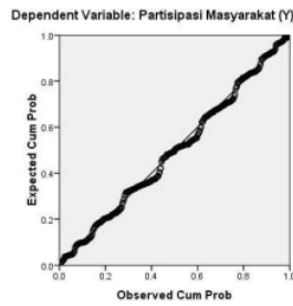
Gambar 1. Normalitas Data
