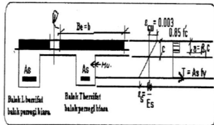
Gambar 7. Diagram regangan-tegangan balok T dan L Semu
