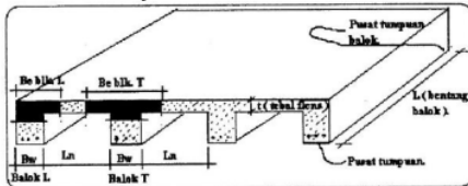
Gambar 4. Notasi pada lebar equivalent Be
