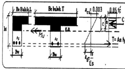
Gambar 6. Diagram tegangan-regangan balok T dan L murni
