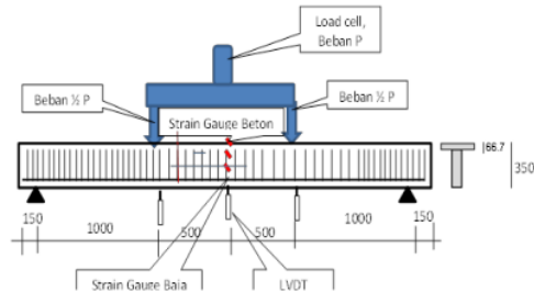
Gambar 9. Sketsa penempatan instrumen pengukuran
