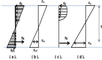
Gambar 1. Distribusi tegangan – regangan penampang balok
