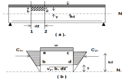
Gambar 2. Mekanisme regangan geser horisontal
