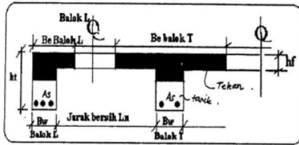
Gambar 3. Bentuk balok T dan L
