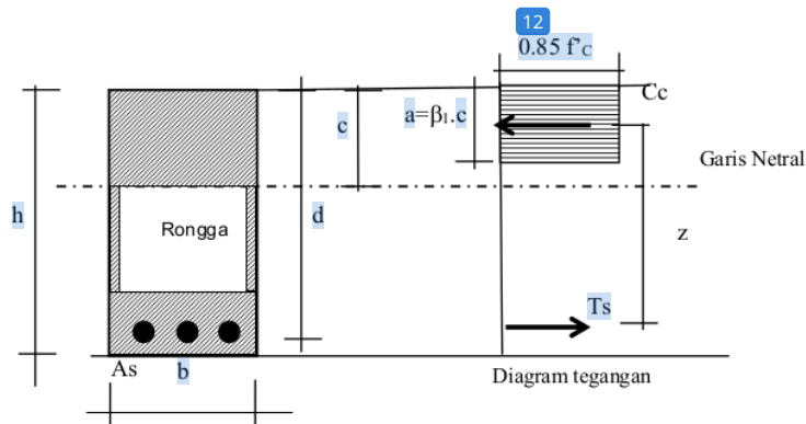
8 Gambar 4. Penampang balok berongga
