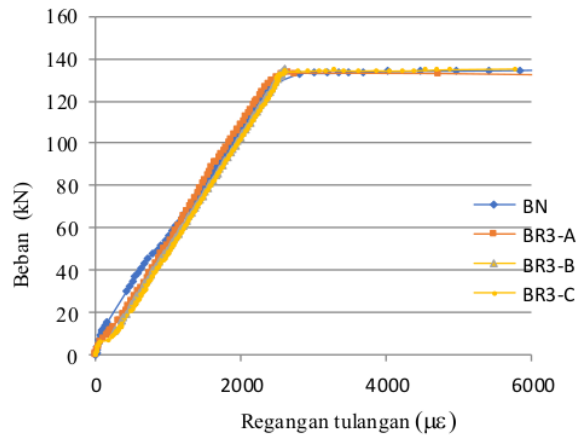
Gambar 10. Hubungan beban dan regangan tulangan
