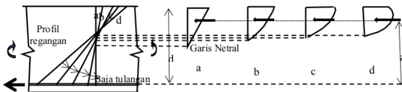
Gambar 1. Diagram regangan dan tegangan balok beton bertulang kondisi seimbang
