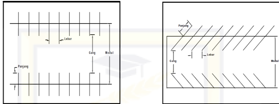
Gambar 2 - 22 Gang dan Modul Sumber: Dirjen Perhubungan Darat
