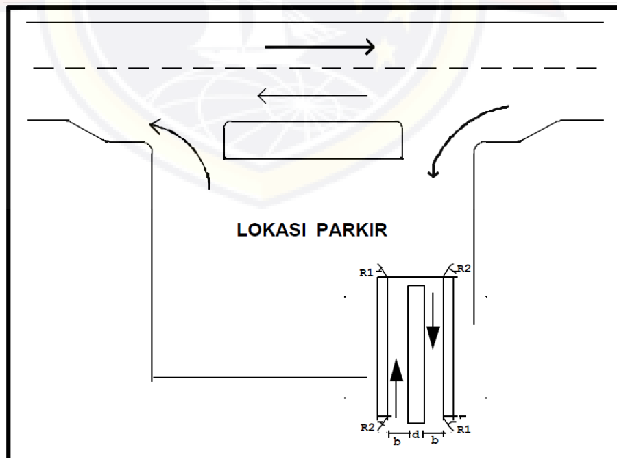
Gambar 2 - 23 Pintu Masuk dan Pintu Keluar Terpisah Sumber: Dirjen Perhubungan Darat
