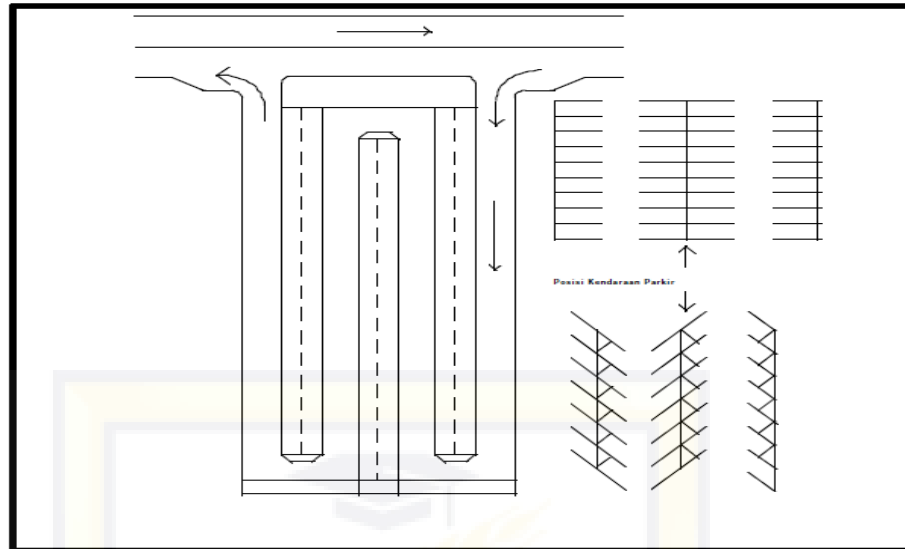
Gambar 2 - 25 Pintu Masuk dan Pintu Keluar Terpisah Pada Satu Ruas Jalan
