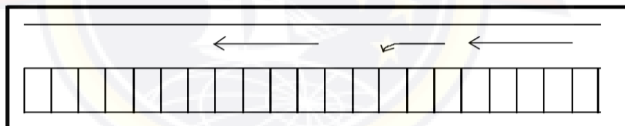
Gambar 2 - 9 Parkir Satu Sisi Dengan Sudut 90^\circ Sumber: Dirjen Perhubungan Darat
