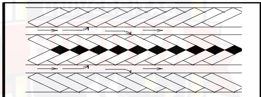
Gambar 2 - 15 Parkir Pulau Dengan Sudut 45^\circ Tipe B Sumber: Dirjen Perhubungan Darat
