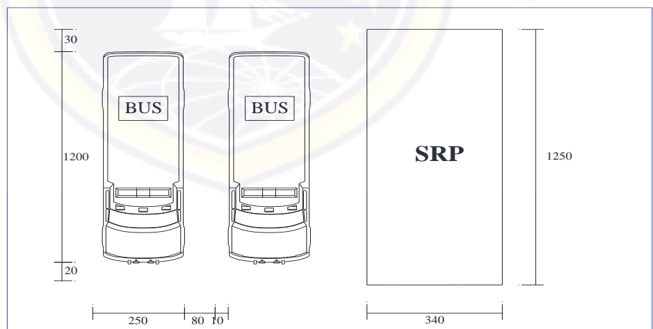
Gambar 2 - 7 Satuan Ruang Parkir (SRP) untuk Bus/Truk
