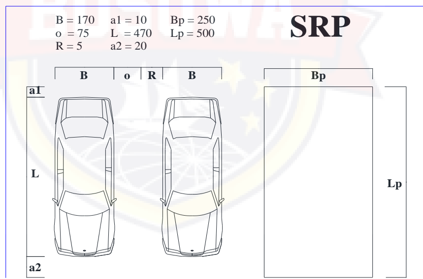
Gambar 2 - 6 Satuan Ruang Parkir (SRP) untuk Mobil Penumpang (dalam cm)
