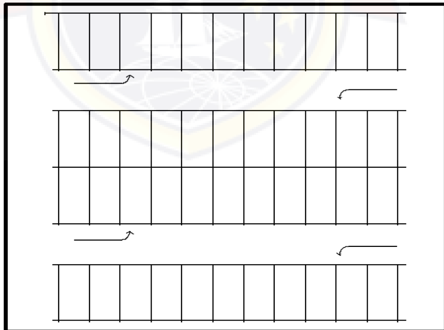
Gambar 2 - 13 Parkir Pulau Dengan Sudut 90^{\circ} Sumber: Dirjen Perhubungan Darat
