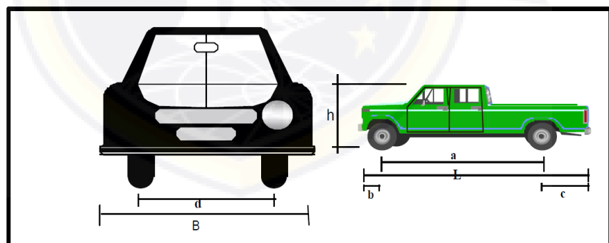
Gambar 2 - 5 Dimensi Kendaraan
