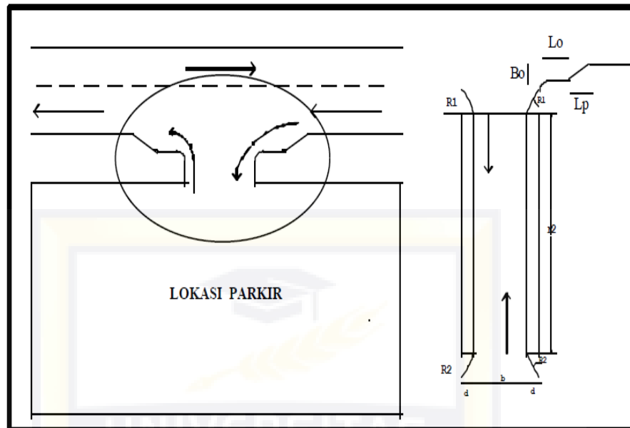
Gambar 2 - 24 Pintu Masuk dan Pintu Keluar Menjadi Satu Sumber: Dirjen Perhubungan Darat
