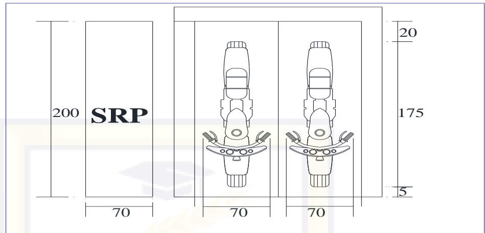
Gambar 2 - 8 Satuan Ruang Parkir (SRP) untuk Sepeda Motor (dalam cm)
