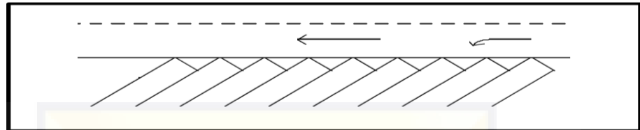
Gambar 2 - 10 Parkir Satu Sisi Dengan Sudut 30^\circ , 45^\circ , 60^\circ Sumber: Dirjen Perhubungan Darat
