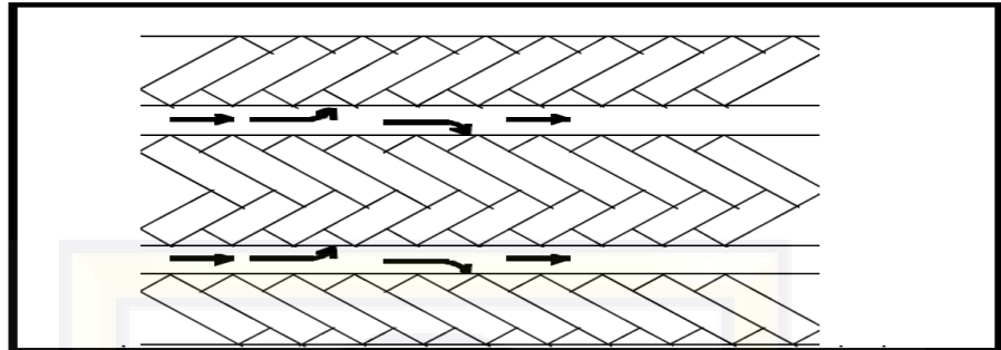
Gambar 2 - 14 Parkir Pulau Dengan Sudut 45^\circ Tipe A Sumber: Dirjen Perhubungan Darat
