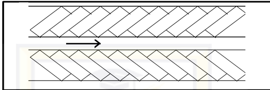
Gambar 2 - 12 Parkir Dua Sisi Dengan Sudut 30^{\circ} , 45^{\circ} , 60^{\circ} Sumber: Dirjen Perhubungan Darat
