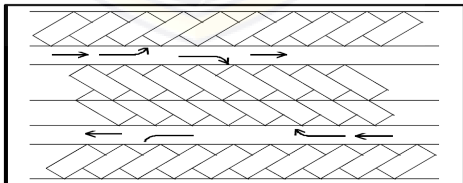
Gambar 2 - 16 Parkir Pulau Dengan Sudut 45^\circ Tipe B Sumber: Dirjen Perhubungan Darat
